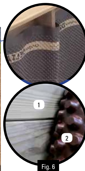
Fig. 6 1- Struttura in legno 2- Rotolo di protezione del drenaggio alveolare di HDPE
