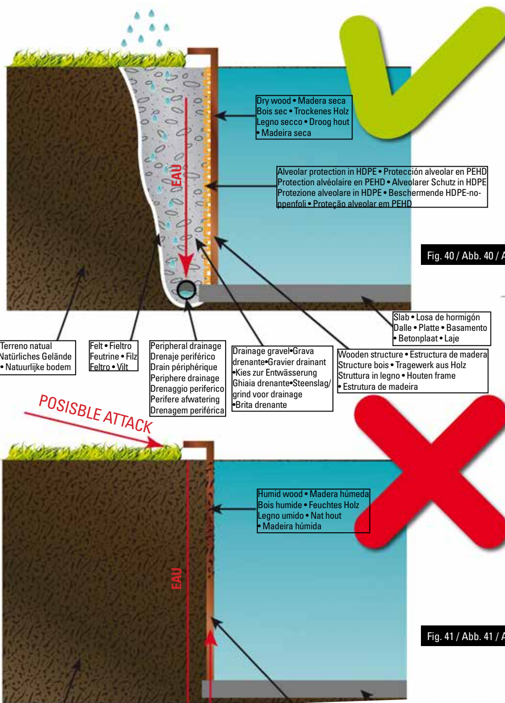
Alveolar protection in HDPE Protección alveolar en PEAD Protection alvéolaire en PEHD Alveolar Schutz in PEHD Protezione alveolare in PEAD Beschermente HDPE-noppenfoli Proteção alveolar em PEAD
